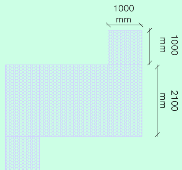
Unité de base à plat pour livraison
